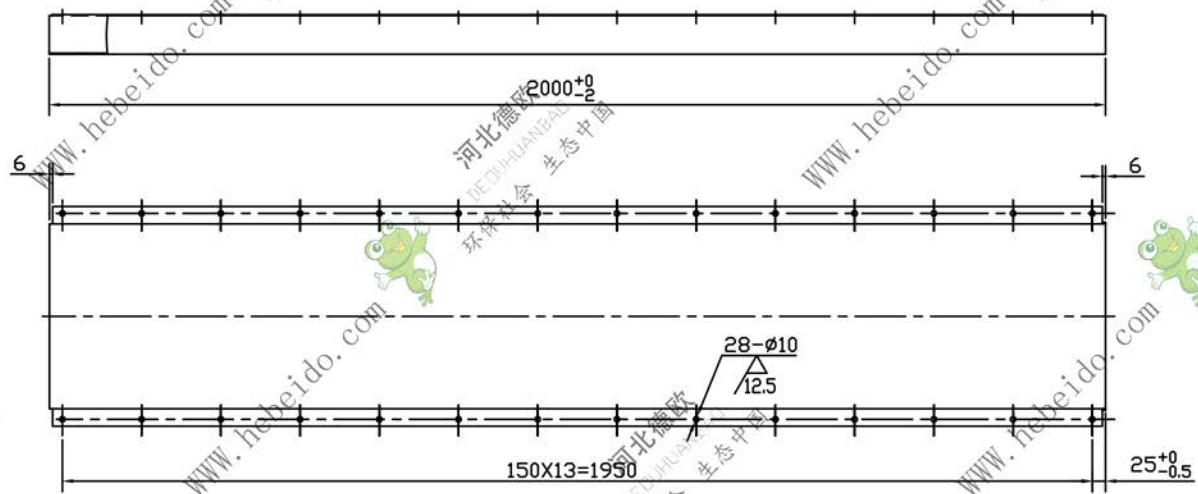
展开图
